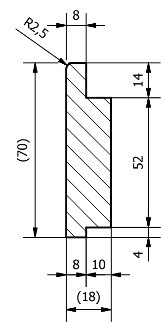
A-A ( 1 : 1.5 )
