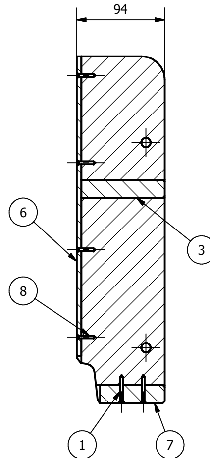
A-A ( 1 : 4 )
